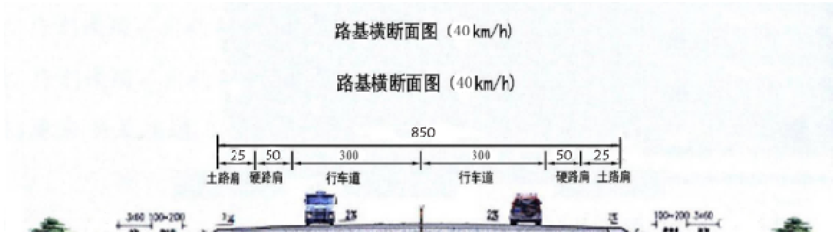
图 2.4-5 连接线路基横断面图（路基宽 7.5m）
