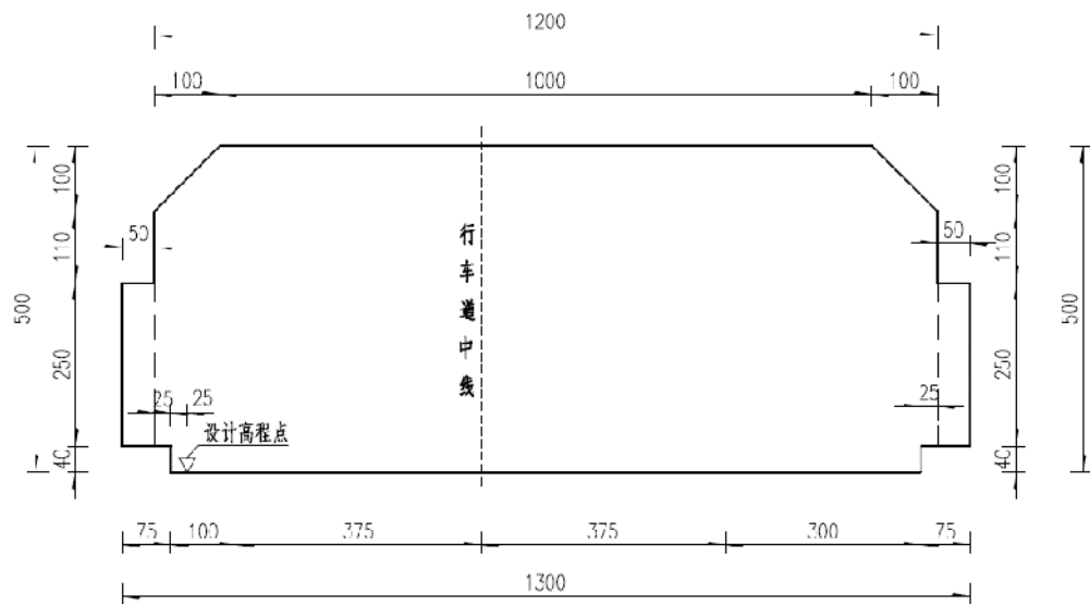
图 2.4-12 短隧道主洞建筑限界图
