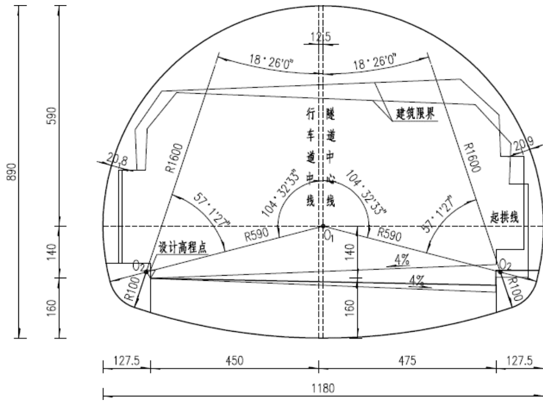
图 2.4-15 中长隧道主洞净空断面图
