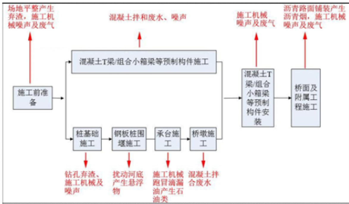
图 2.5-5 大桥施工工序及产污节点
