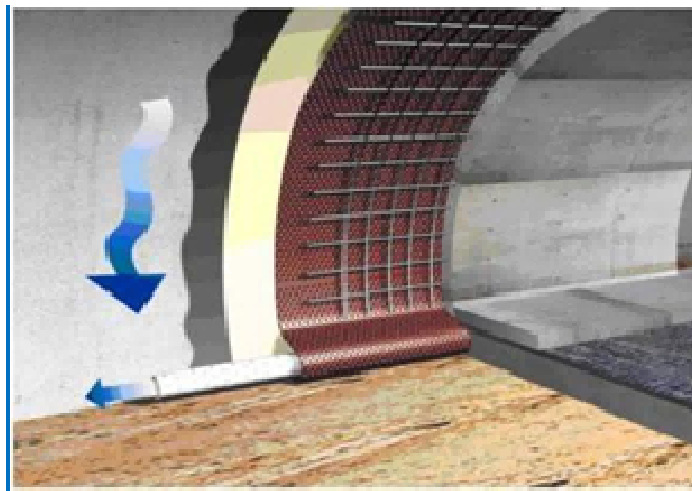
图 2.4-17 主线隧道防排水设计图
