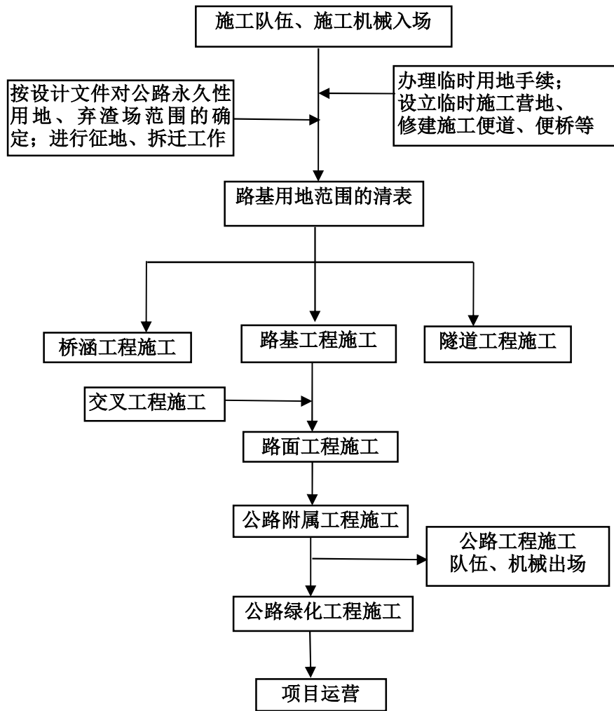
图 2.4-19 工程施工流程图
