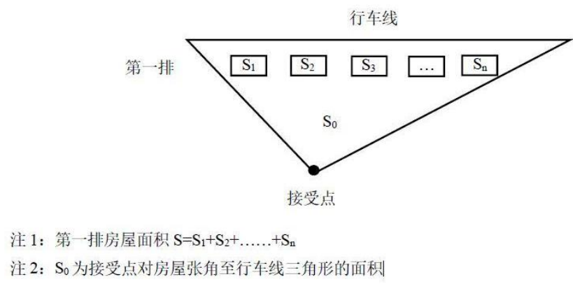
图 4.4-3 建筑物引起的衰减量计算示意图
