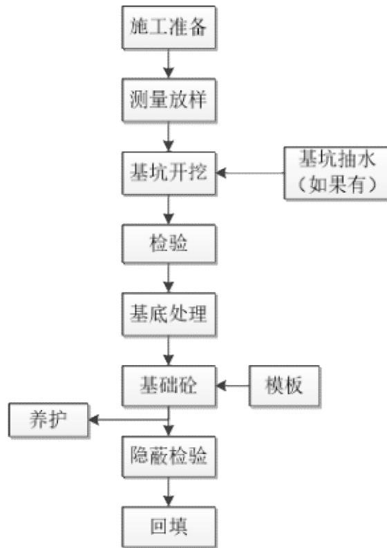
图 2.4-20 明挖扩大基础施工工艺流程
