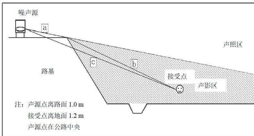
图 4.4-4 声程差 \delta 计算示意图
