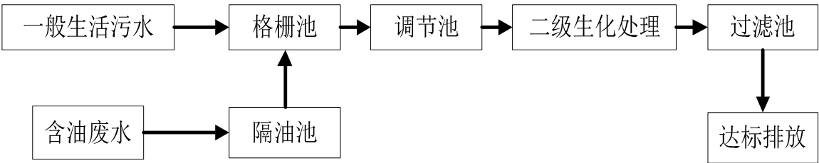
图 5.1-1 污水处理工艺流程
