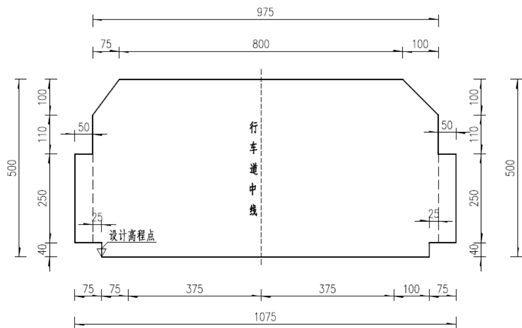
图 2.4-14 中长隧道主洞建筑限界图
