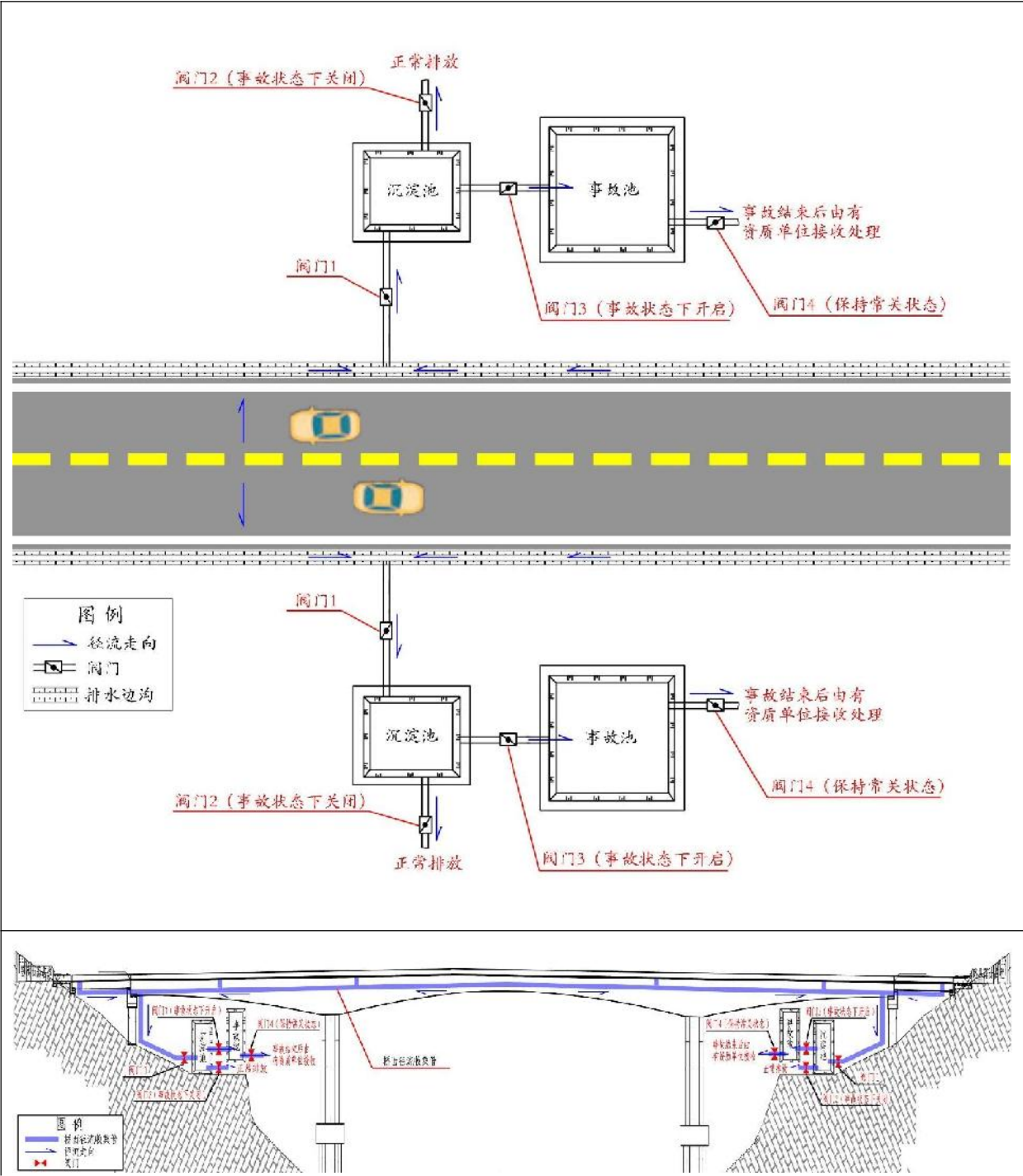
图 5.5-1 典型桥面径流收集系统横断面和实物图
