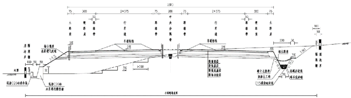
图 2.4-2 26.0m 宽，整体式路基标准横断面图
