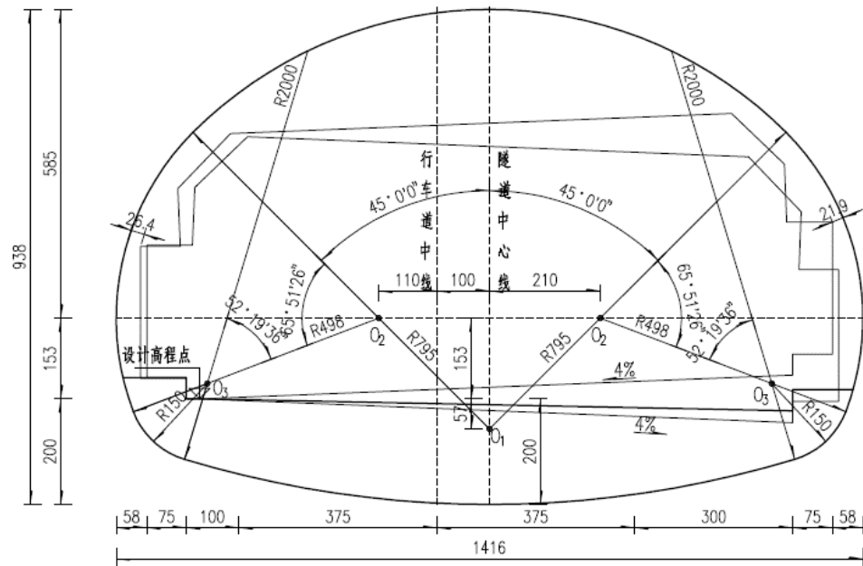
图 2.4-13 短隧道主洞净空断面图
