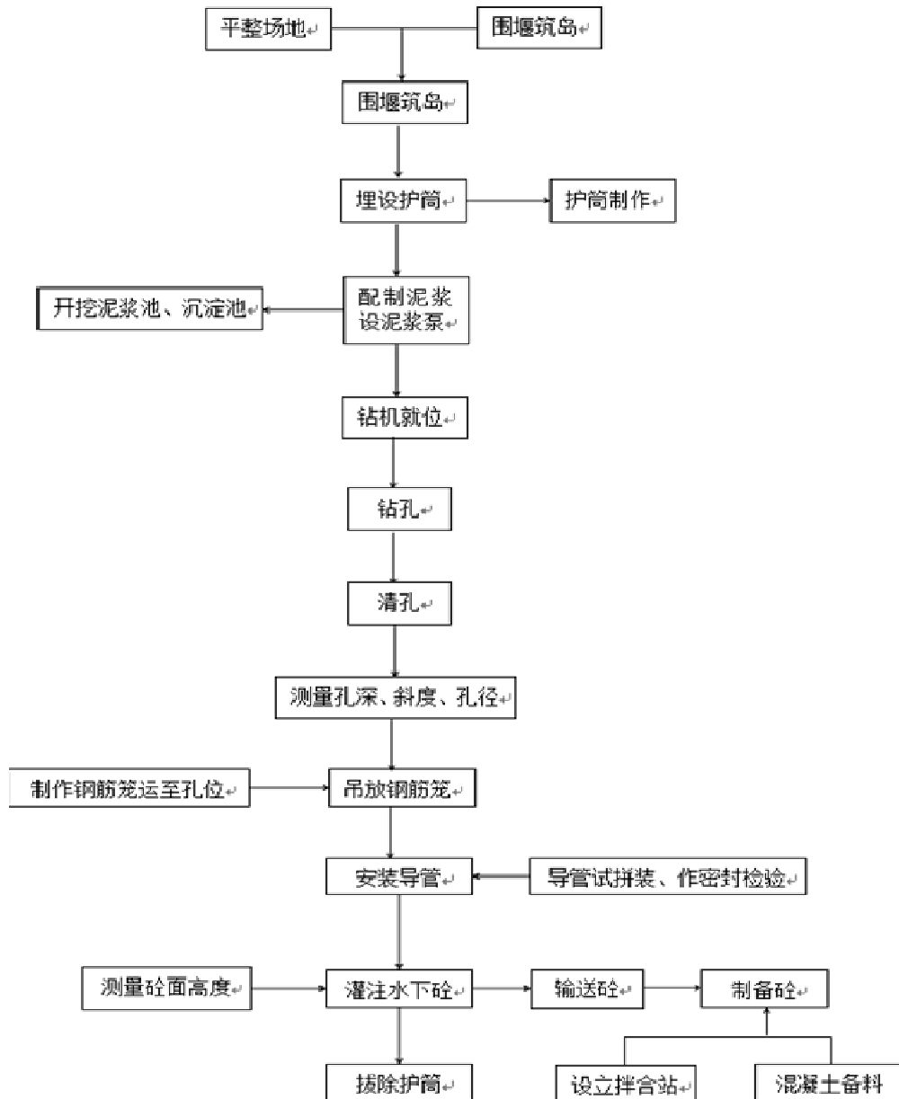
图 2.4-21 钻孔灌注桩基础施工工艺流程图
