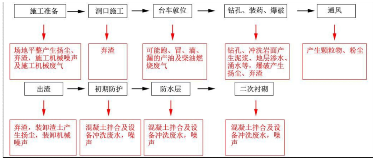
图 2.5-6 隧道施工工序及产污节点
