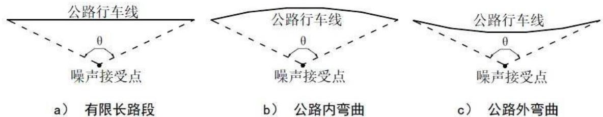
图 4.4-1 预测点到有限长路段两端的张角
