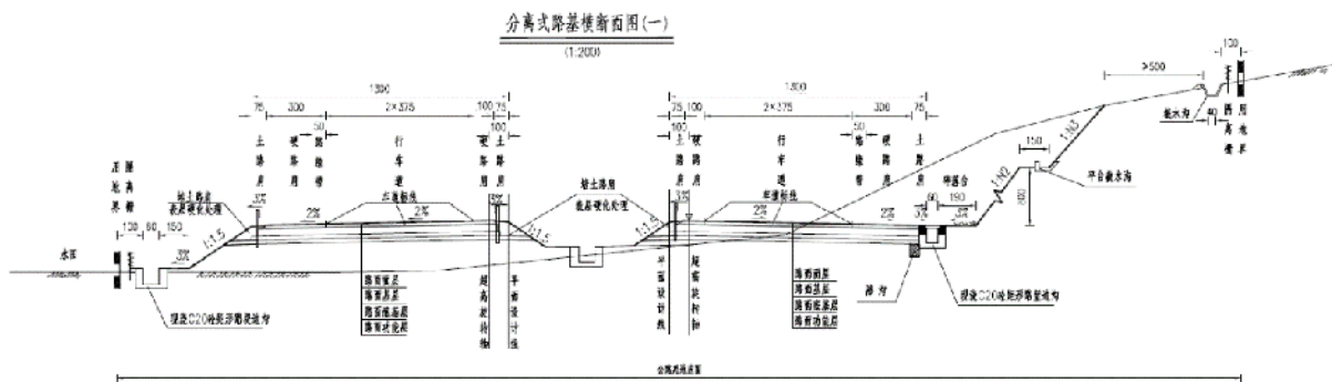
图 2.4-3 13.0m 宽，分离式路基标准横断面图
