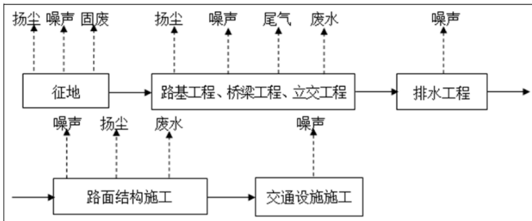
图 2.5-7 一般路段施工工序及产污节点
